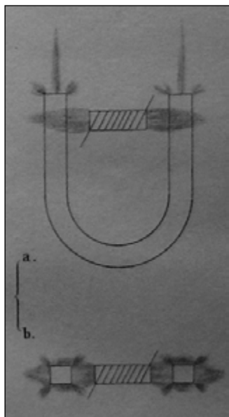
Рис.7. Обычный подковообразный магнит и бруско- вый электромагнит с обмоткой из медной проволоки в положении один в другом. Вид сбоку (а) и вид сверху (b).
