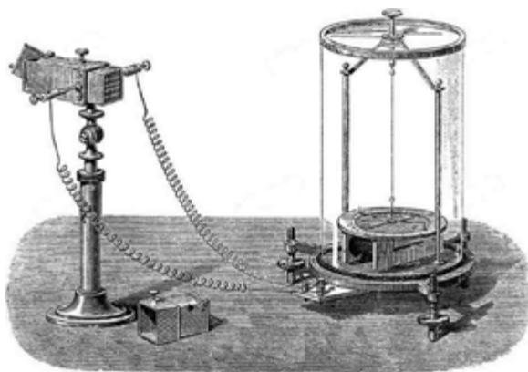
Термоскоп Нобили с гальванометром
